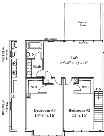
LEFT END UNIT
